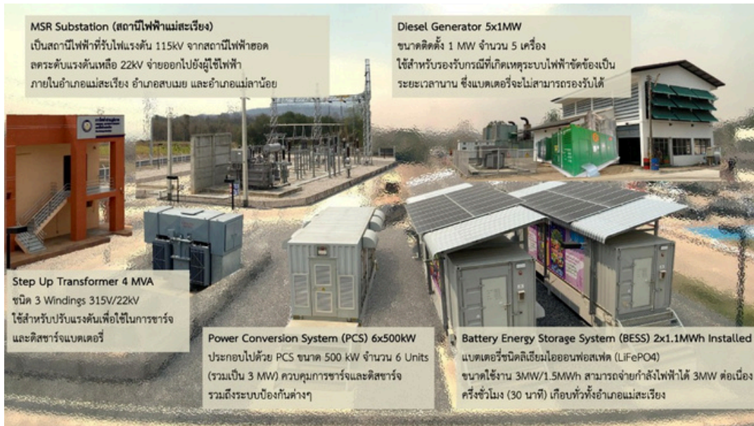
โครงข่ายไฟฟ้าขนาดเล็กมาก (Microgrid) อำเภอแม่สะเรียง จังหวัดแม่ฮ่องสอน ที่มา: www.temca.pea.co.th
